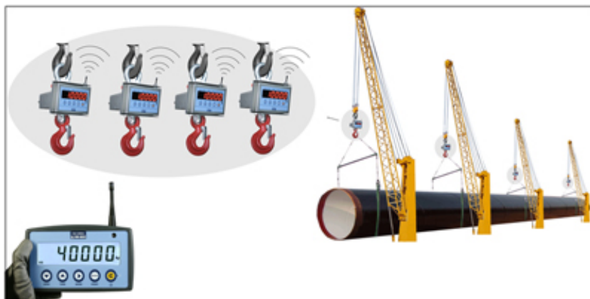
DFWPM : Répétiteur de poids multi balances.
